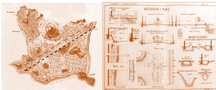
PLANTA DO PROJETO NOVO ARRABALDE (VITÓRIA, ES); DETALHES E CORTES DO PROJETO PARA AVENIDAS E RUAS; TRACEJADO EM PRETO, A AVENIDA LEITÃO DA SILVA, PRAIA DO SUÁ. PROJETO DE AUTORIA DO ENGENHEIRO FRANCISCO SATURNINO DE BRITO, 1896. FONTE: TEIXEIRA JUNIOR, CARLOS. O NOVO ARRABALDE.VITÓRIA: PMV, SECRETARIA MUNICIPAL DE CULTURA E TURISMO, 1996.
